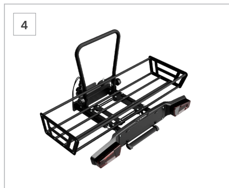
4 Cestino per portacarichi posteriore SEGSYA7200
